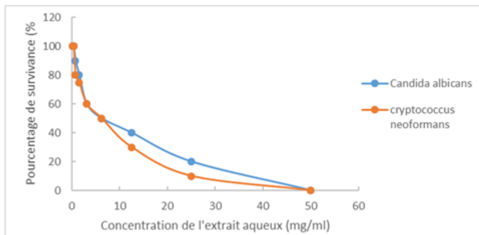
Figure 2 : Courbes de sensibilité de l'extrait aqueux de Hugonia platysepala
